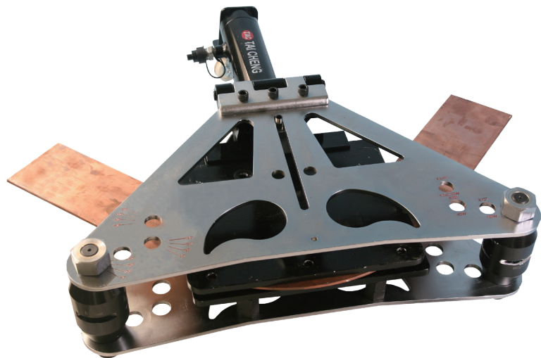
CB-125 二合一平立彎工具 (單迴路)
