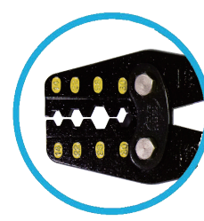
TP-38HB/HM :六角
